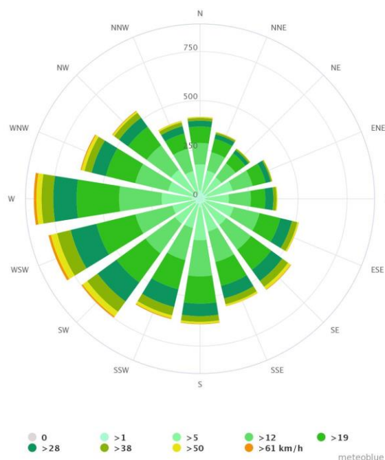
Rys. 3. Róża wiatrów dla Suwałk w latach 1961 – 1995
